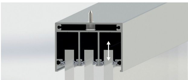
Höhenausgleich
